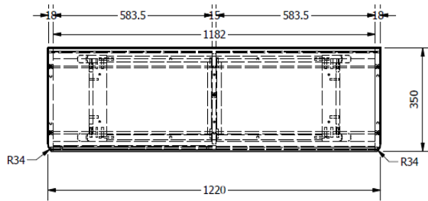
TOP VIEW TAMPAK ATAS
