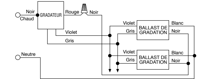
Figure 2 – câblage 3 voies
