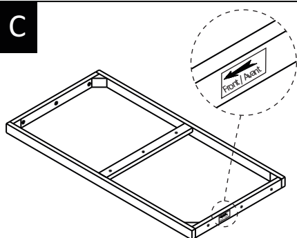
BOTTOM FRAME QTY 1
