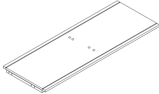
BOTTOM (1 pc)
