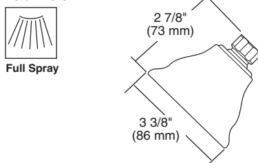
H777▲
