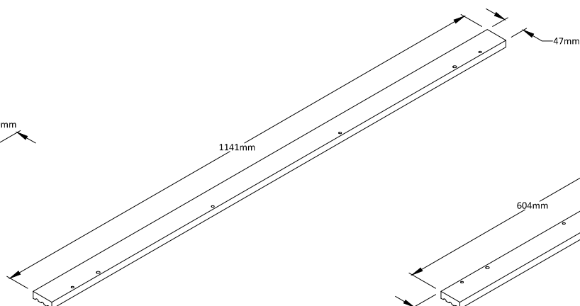
47 UPPER RAIL Qty:2
