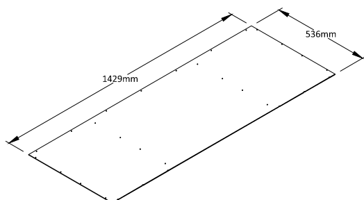
52 UPPER BACK PANEL Qty:1
