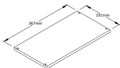
49 ADJUSTABLE SHELF Qty:2
