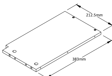
50 UPPER LEFT BOTTOM Qty:1
