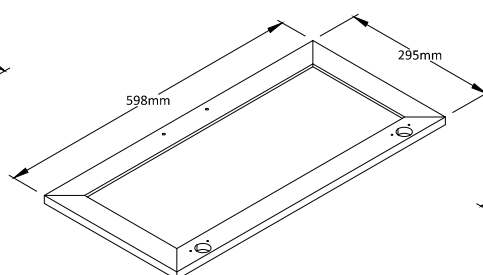
53 UPPER DOOR Qty:2
