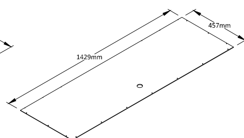
54 UPPER BACK PANEL Qty:1
