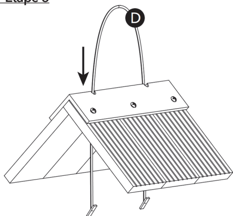
Step 5 / Paso 5 / Étape 5
