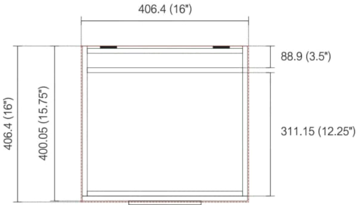
. TOP ELEVATION
