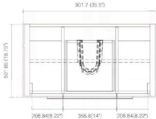
TOP ELEVATION
