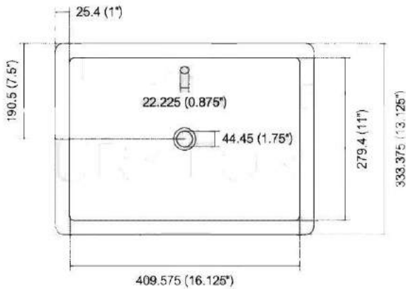
TOP ELEVATION
