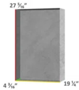
Cutout Dimensions
