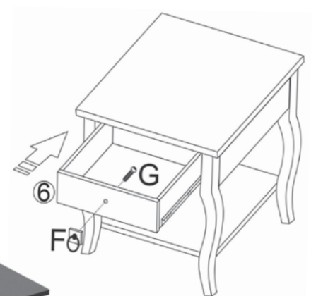
Assembled Table Table assemblée Mesa ensamblada
