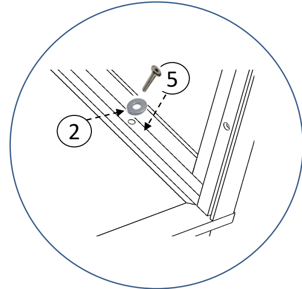
DETAIL Y
