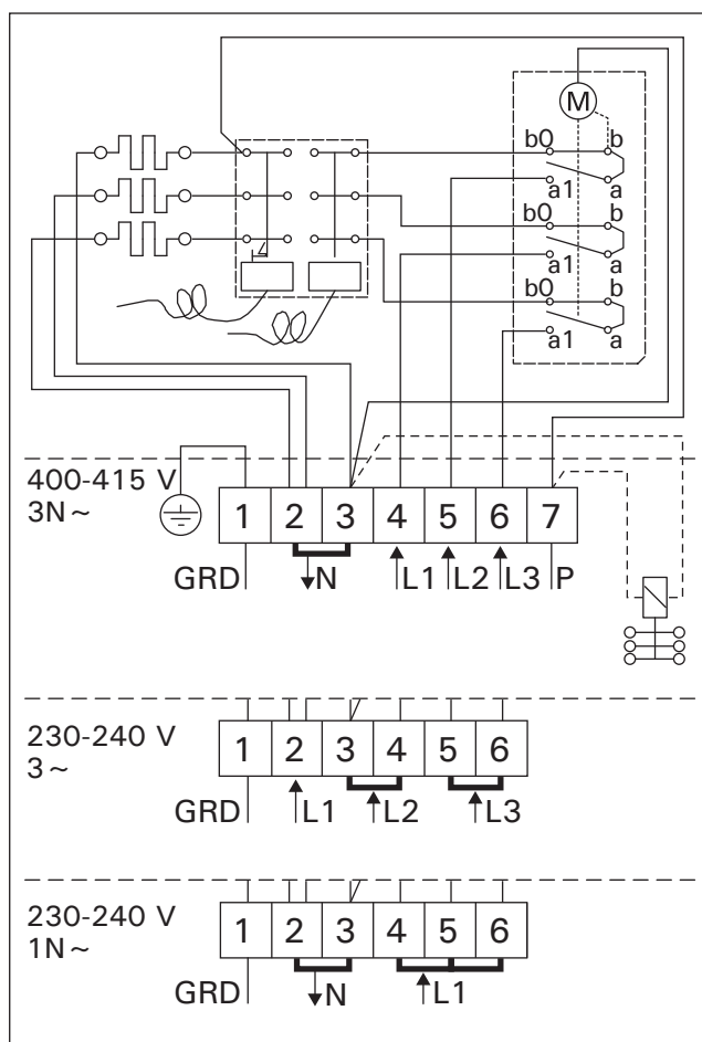
10. zīm. Elektrības pievienošana BC krāsnij 10 pav. BC krosnelių elektrinė schema
