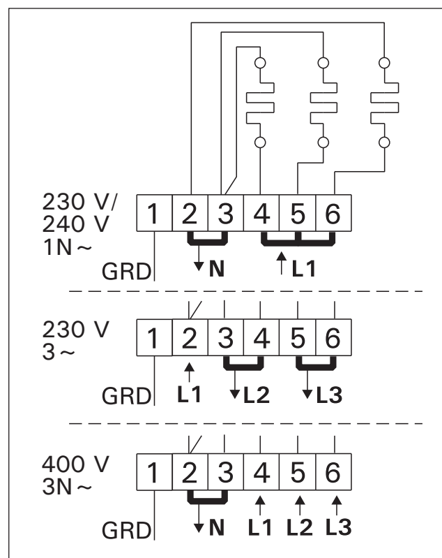
11. zīm. Elektrības pievienošana BC-E krāsnij 11 pav. BC-E krosnelių elektrinė schema
