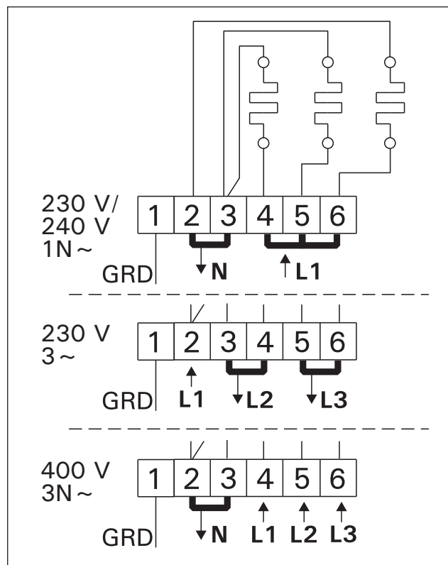
Kuva 11. BC-E-kiukaan sähkökytkennät Bild 11. BC-E-aggregatets elinstallationer
