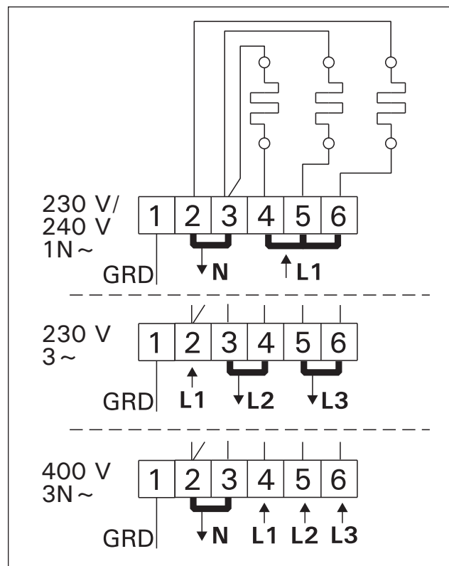
Figura 11. Conexiones eléctricas (BC-E) Фигура 11. Електрически връзки на модел BC-E
