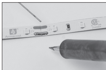
Raccordement du ruban
