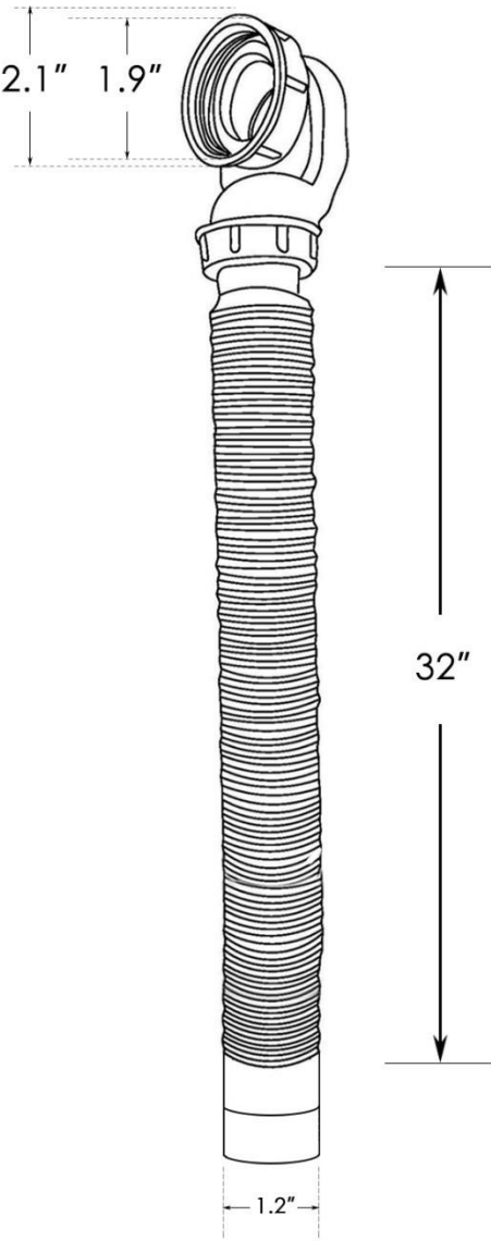
Imagen 3: Conjunto de drenaje PVC
