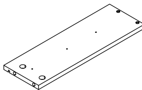
(H) DRAWER LEFT PANEL Qty:2
