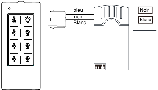
TÉLÉCOMMANDE(1PCS)
