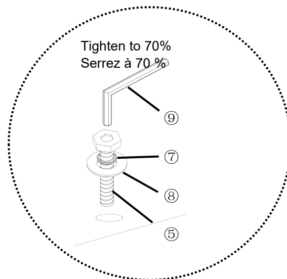
Right Arm/Accoudoir droit(D)
