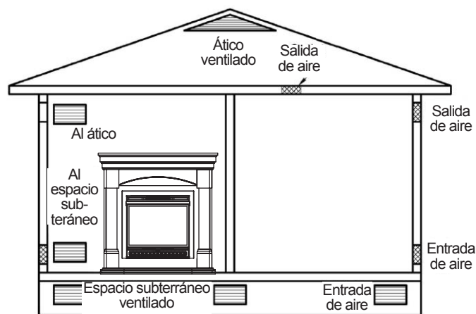
Fig. 5: aire de ventilación del exterior
