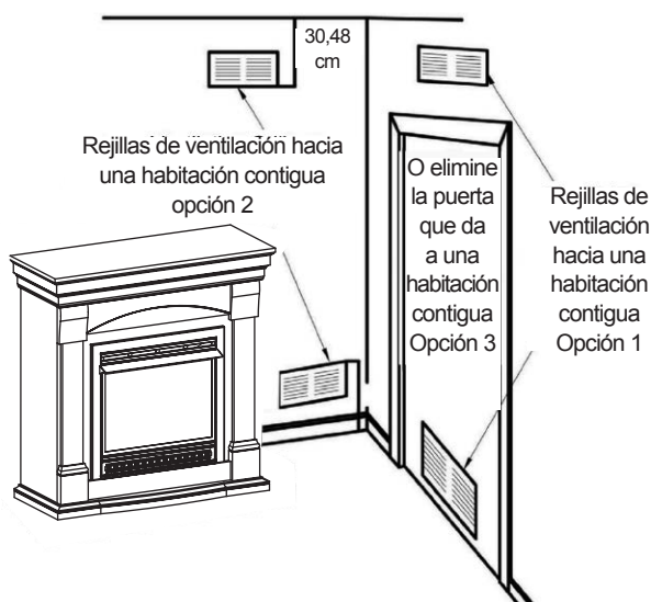
Fig. 4: aire de ventilación del interior del edificio
