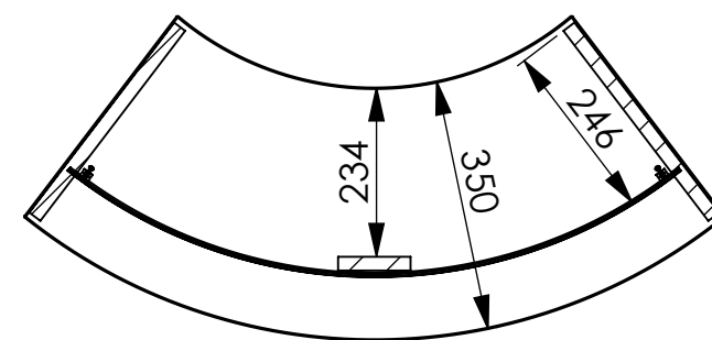
COUPE A-A ECHELLE 1 : 11.5
