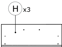
CS3759 499x189x22mm
