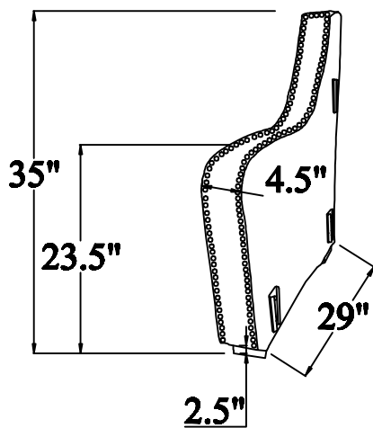
ARM
