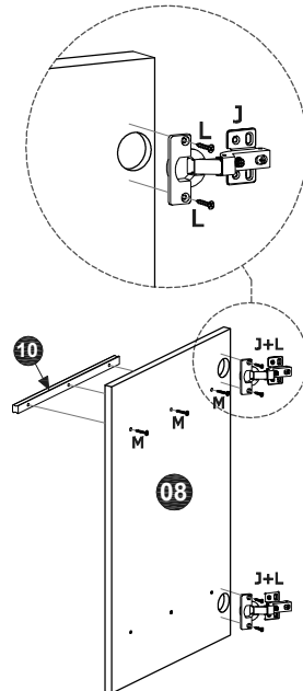
DETAIL 4 / DÉTAIL 4
