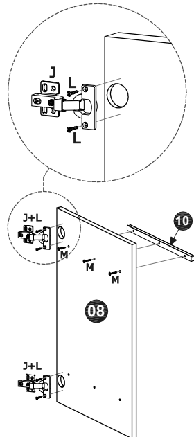
DETAIL 3 / DÉTAIL 3
