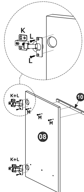
DETAIL 5 / DÉTAIL 5
