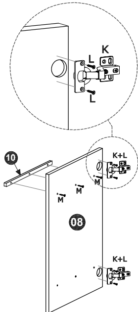
DETAIL 2 / DÉTAIL 2
