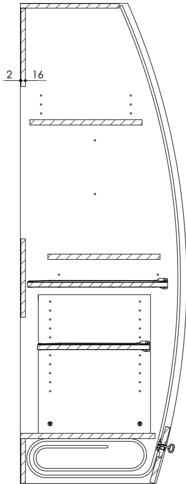
COUPE B-B ECHELLE 1 : 8
