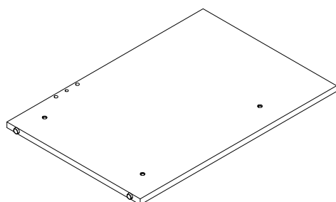
CABINET LEFT SIDE PANEL Qty:1
