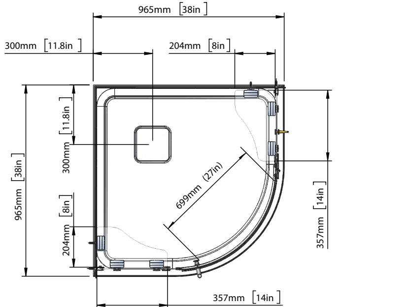
Top View - Vue de dessus- Vista superior
