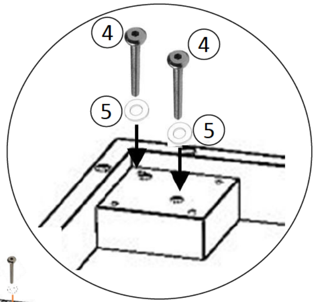
DETAIL Y
