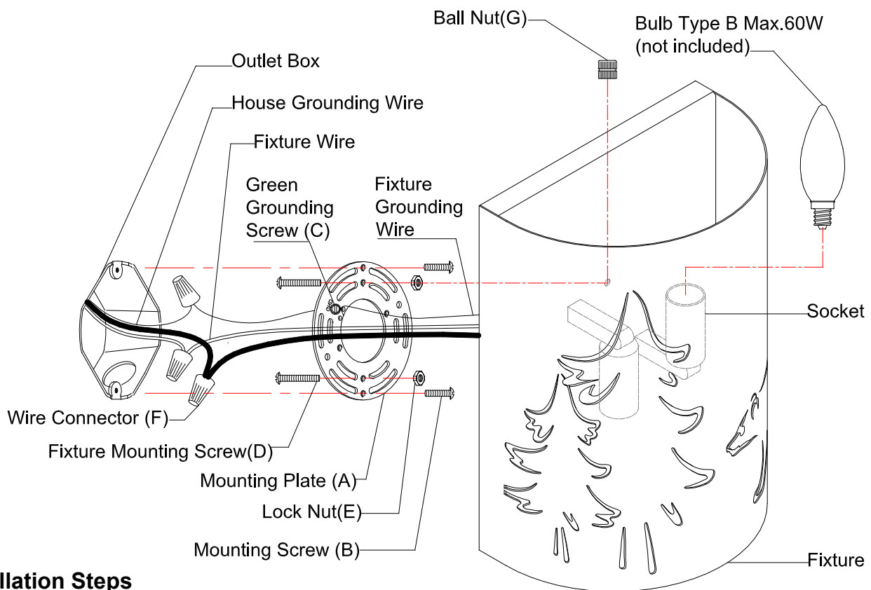
Fixture Mounting Screw (D)
