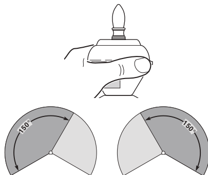
Rotation du capteur pour modifier la zone de couverture
