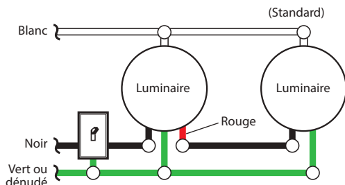
Diagramme de câblage 1
