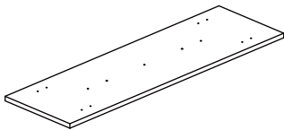
29 (1090*330*18mm x1)
