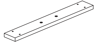
24 (500*70*18mm x2)
