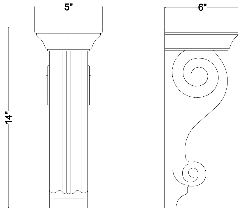
ITEM NUMBER:COR05X06X14SA 5"W x 6"D x 14"H Salem Corbel
